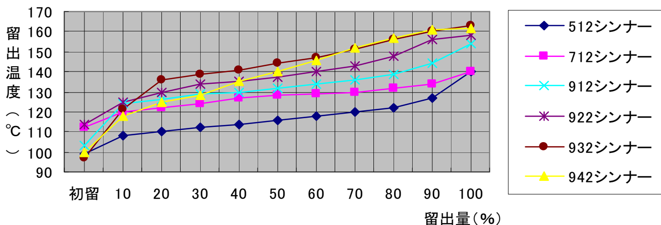
蒸留曲線
