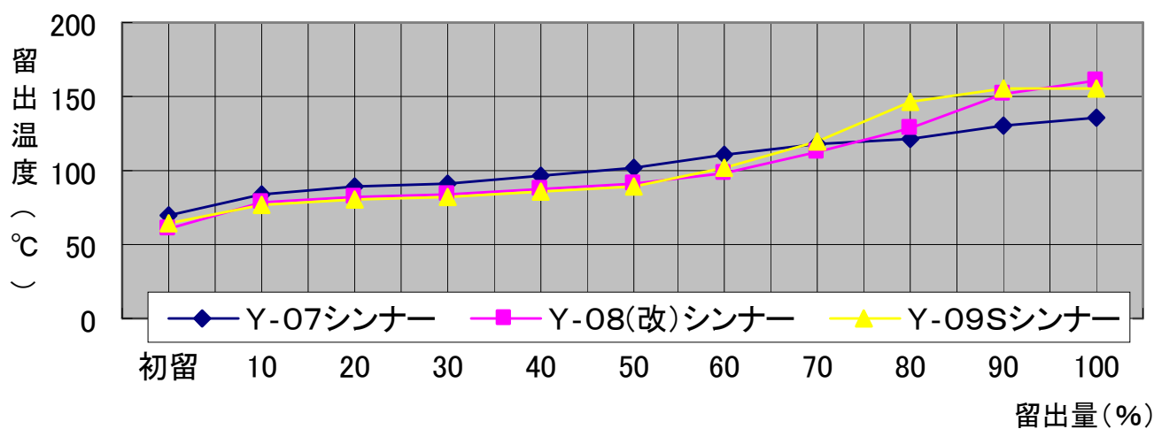
蒸留曲線
