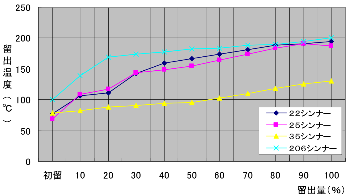
蒸留曲線
